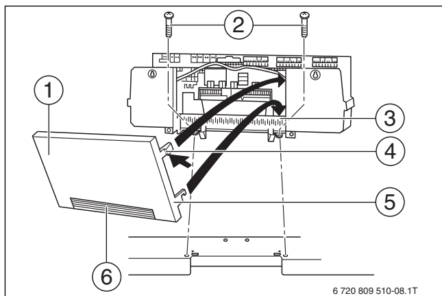
Рис. 25 Крепление Logamatic 4000
