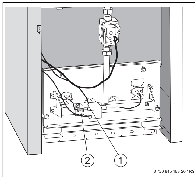
Рис. 38 Удаление защиты от прикосновения
