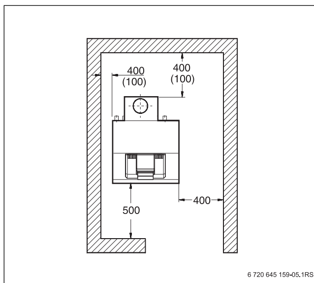
Рис. 7 Рекомендуемые расстояния от стен (размеры в мм, в скобках указаны минимальные размеры)
