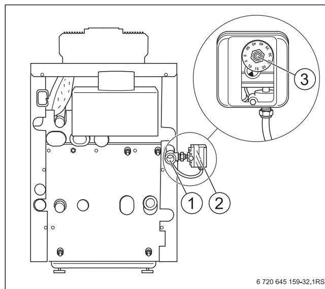
Рис. 55 Установка реле контроля давления газа
