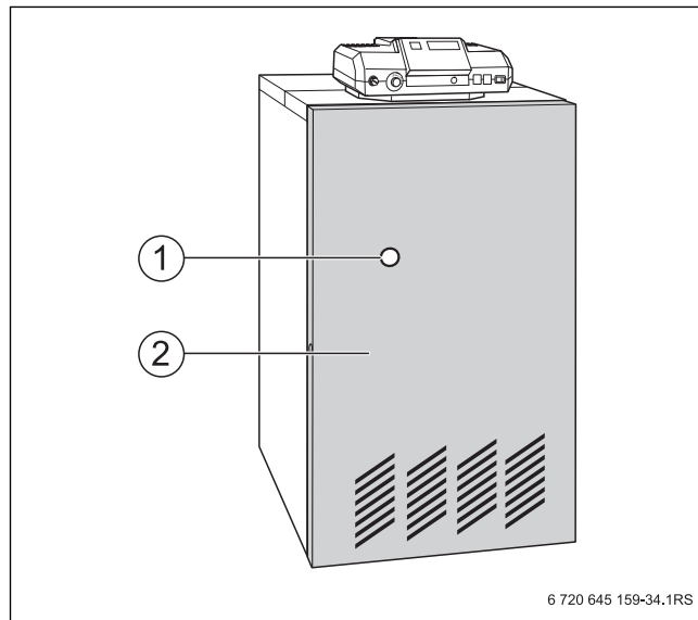
Рис. 61 Устранение неисправностей горелки
