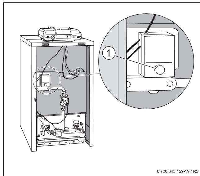
Рис. 35 Кнопка подавления помех/сигнальная лампа
