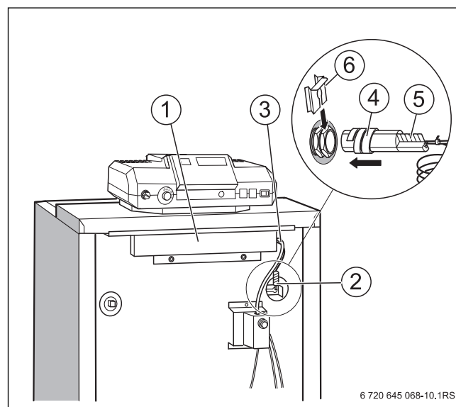
Рис. 21 Установка комплекта датчика температуры
