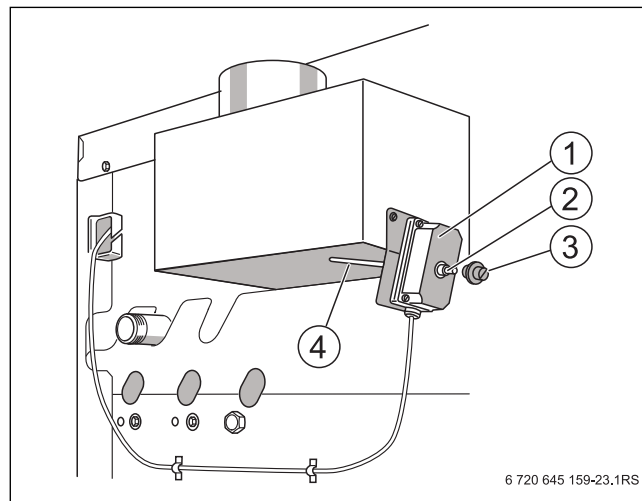
Рис. 41 Проверка устройства контроля дымовых газов AW 10
