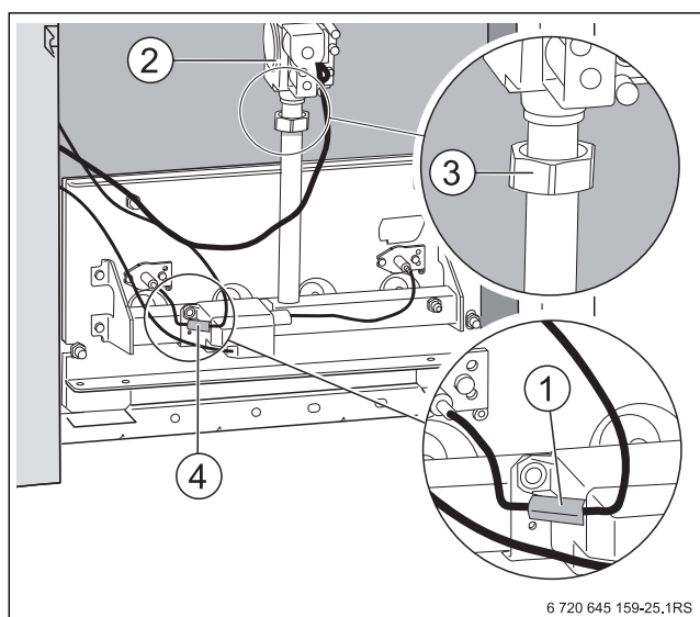
Рис. 49 Демонтаж горелки
