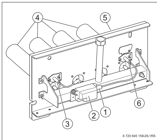
Рис. 53 Чистка горелки
