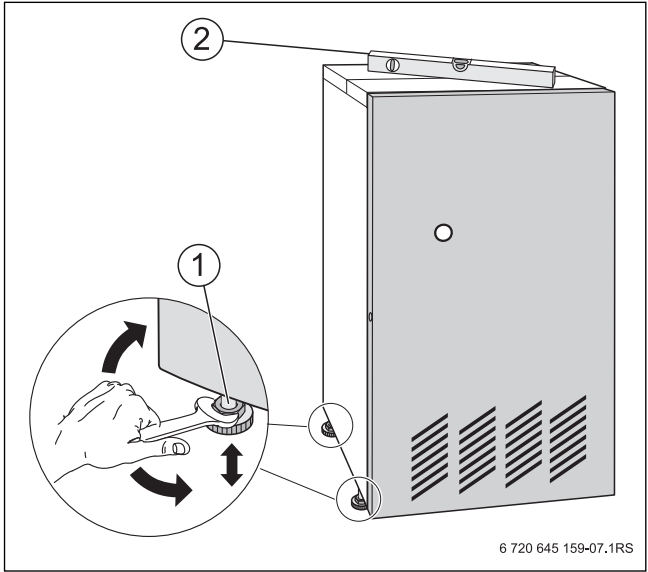
Рис. 9 Выравнивание котла
